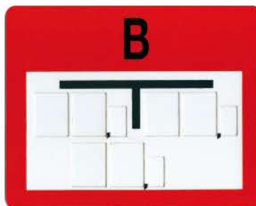
4066 B Löschwasserbrunnen mit unmittelbarem Kraftspritzen-Anschluss, 200 x 250 mm
